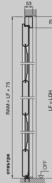
Странична врата от масивна дървесина Монтаж в отвора
