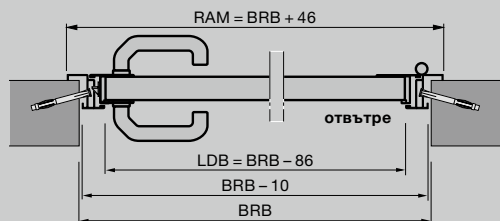
Странична врата с алуминиева ъглова каса, профил тип 3 Външен ограничител
