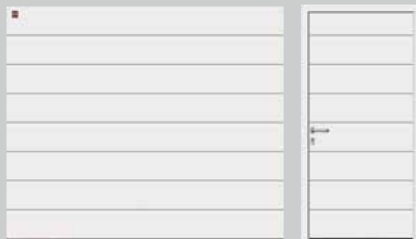
Обшивка на М-линии (LPU, LTE), транспортно бяло RAL 9016
