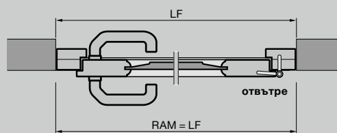
Странична врата от масивна дървесина Монтаж в отвора
